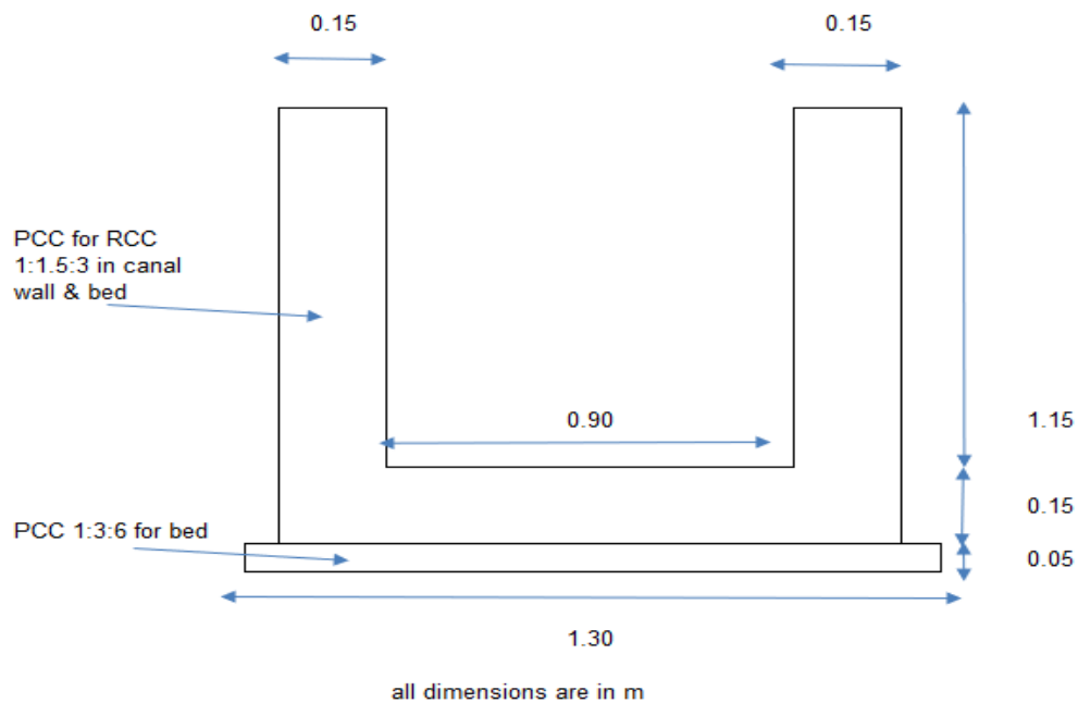
Fig: Canal Section
