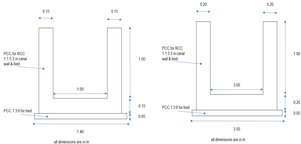
Fig: Canal Section
